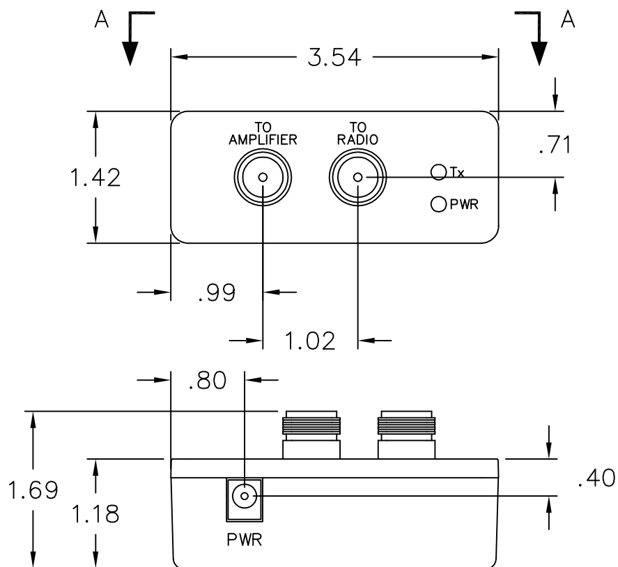
VIEW A-A
