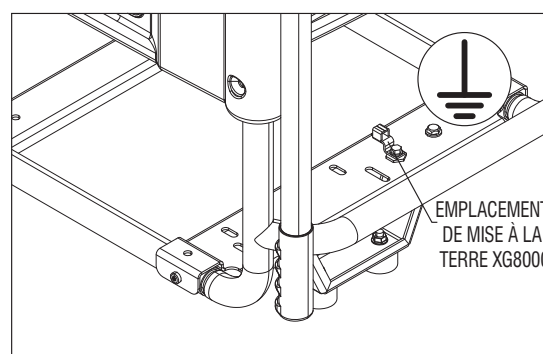
Schéma 6 – Emplacement de mise à la terre du générateur
