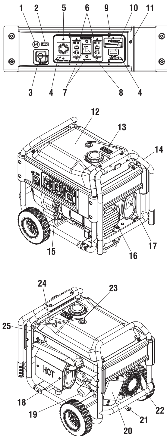
Schéma 3 – Emplacements du générateur
