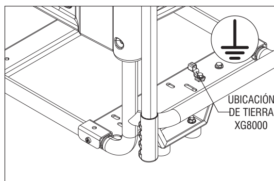
Figura 6 – Ubicaciones de la tierra del generador
