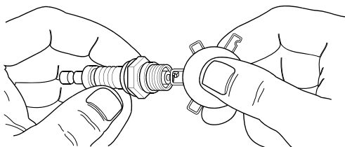
Figura 12 - Espaciamento de la bujía
