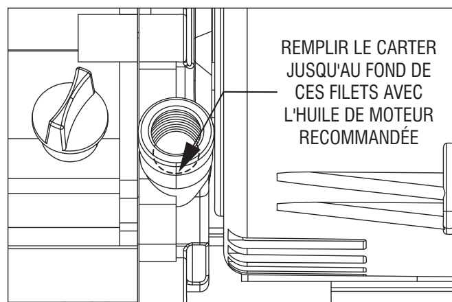
Schéma 8 – Niveau d'huile
