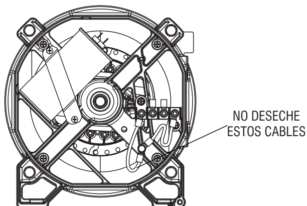
Figura 7 – Conexión a tierra de neutro a marco
