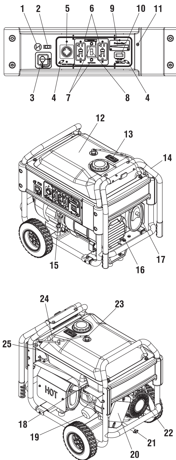
Figura 3 – Ubicaciones del generador
