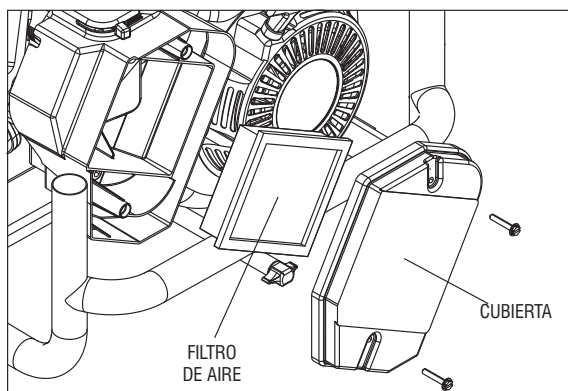
Figura 13 - Filtro de aire
