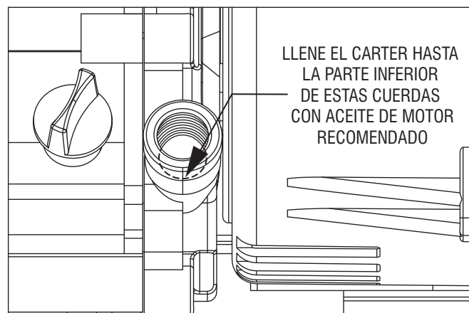
Figura 8 – Nivel de aceite
