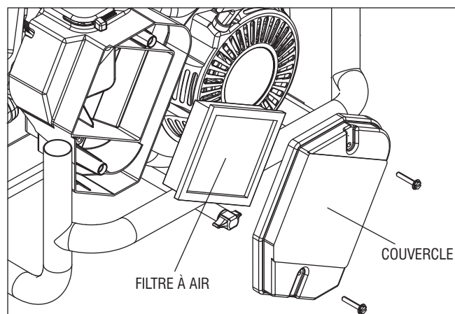
Schéma 13 – Filtre à air
