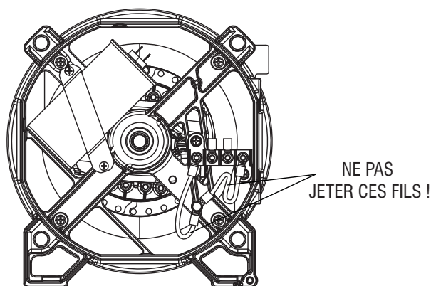
Schéma 7 – Mise à la terre du conducteur neutre au châssis
